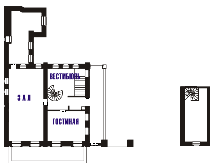
Рис. 2. План первого этажа и мезонина особняка на Чаплыгина 36 (из: [2, стр. 152], надписи на плане поставлены мной - З. Х.)
