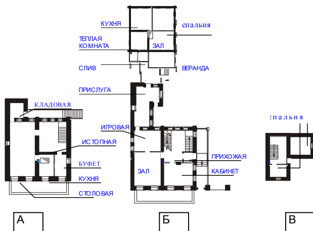
Рис. 5. План подвала (А), первого этажа (Б) и мезонина (В) особняка на Чаплыгина 36. Реставрация.
