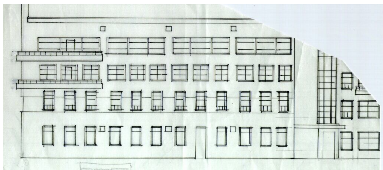
Рис. 5. Фасад дома на Красном проспекте 13. Эскиз проекта стилового реконструкции. Предложение автора статьи.
