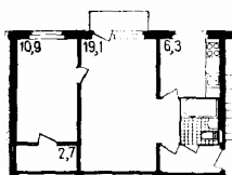
Рис.2. Так называемые “экономичные планировки” квартир для посемейного заселения. Типовые проекты 1957-1963 годов. Серия 1-335. План двух-комнатной квартиры из рядовой секции. Достижением можно считать увеличение как общей, так и жилой площадей квартиры по сравнению с 1920-ми годами.
